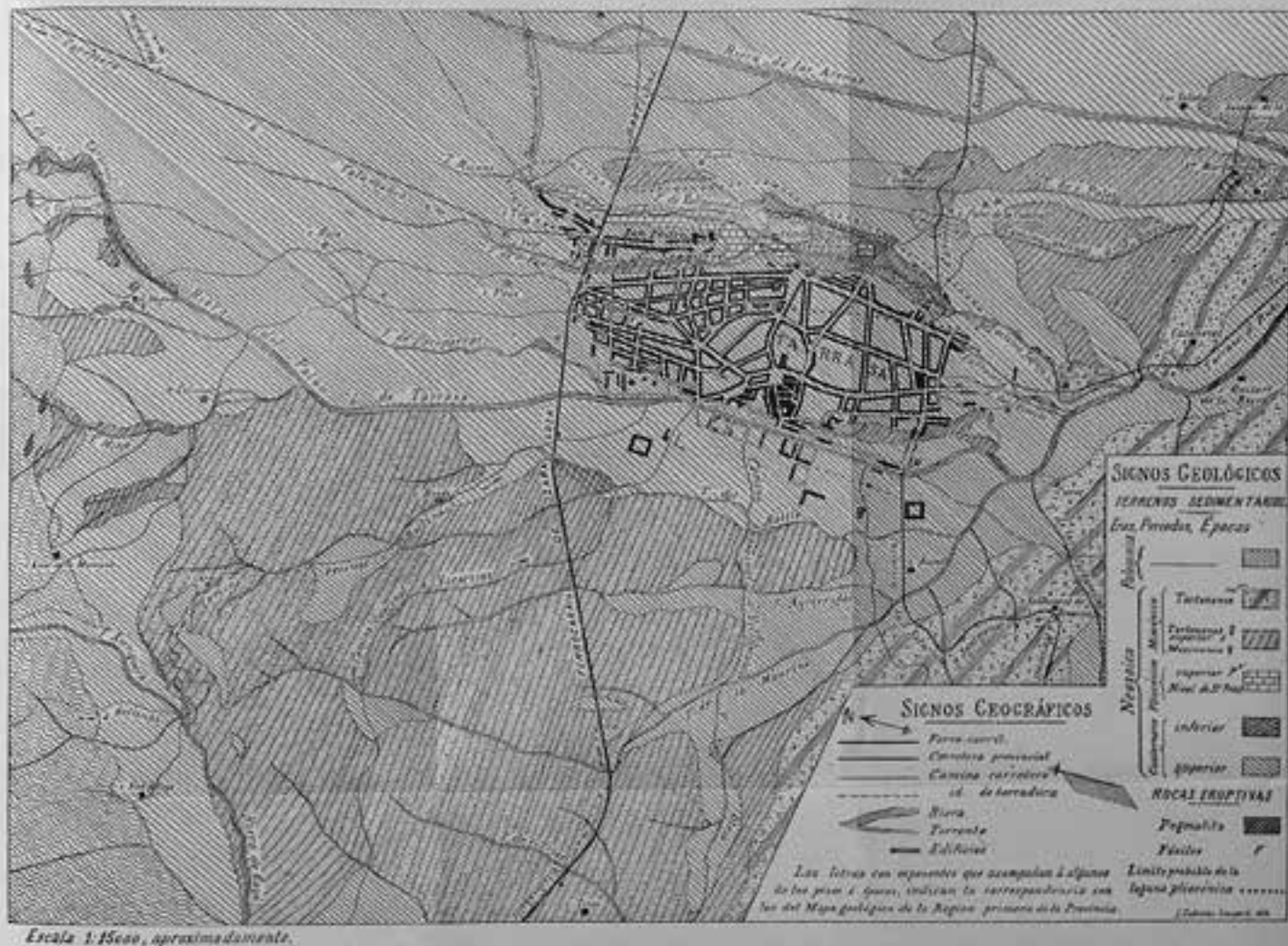
Fig. 12.—MAPA GEOLÓGICO DE LOS ALREDEDORES DE TERRASA, por D. Domingo Palet.
